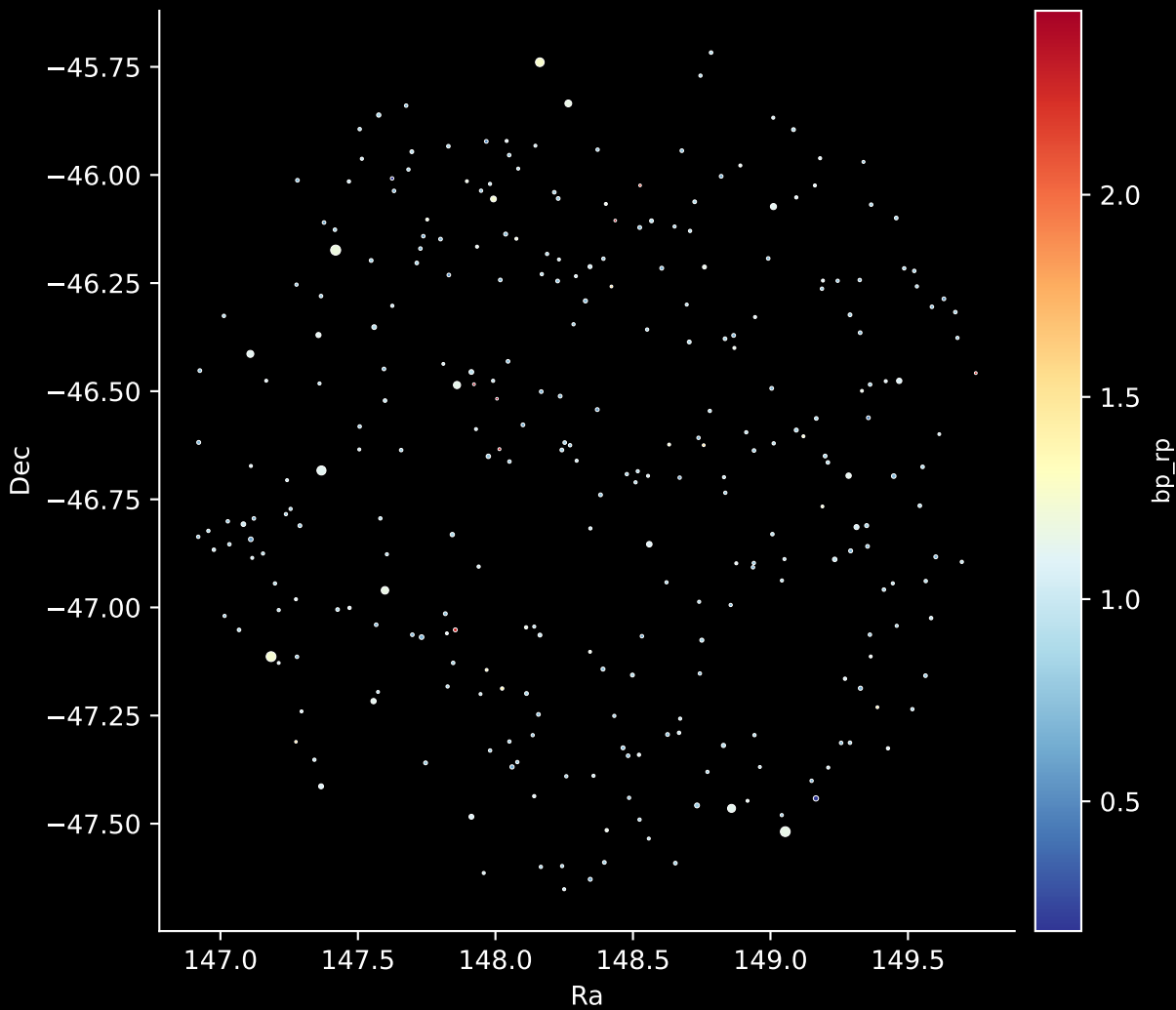
GALAH DR4 Field: [6883] Stars: 294
