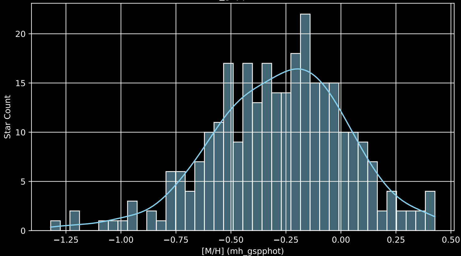
GALAH DR4 Field: [6883] [M/H] (mh_gspphot) (n= 294)
