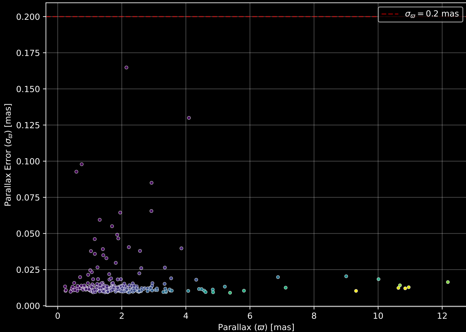
GALAH DR4 Field: [6883] Parallax Quality (n= 294)
