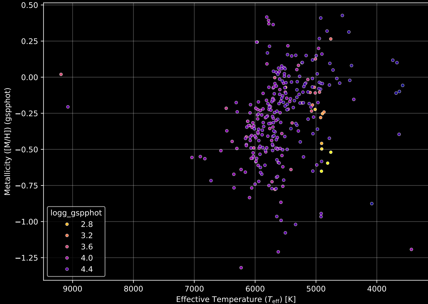
GALAH DR4 Field: [6883] Stellar Population Parameters (n= 294)
